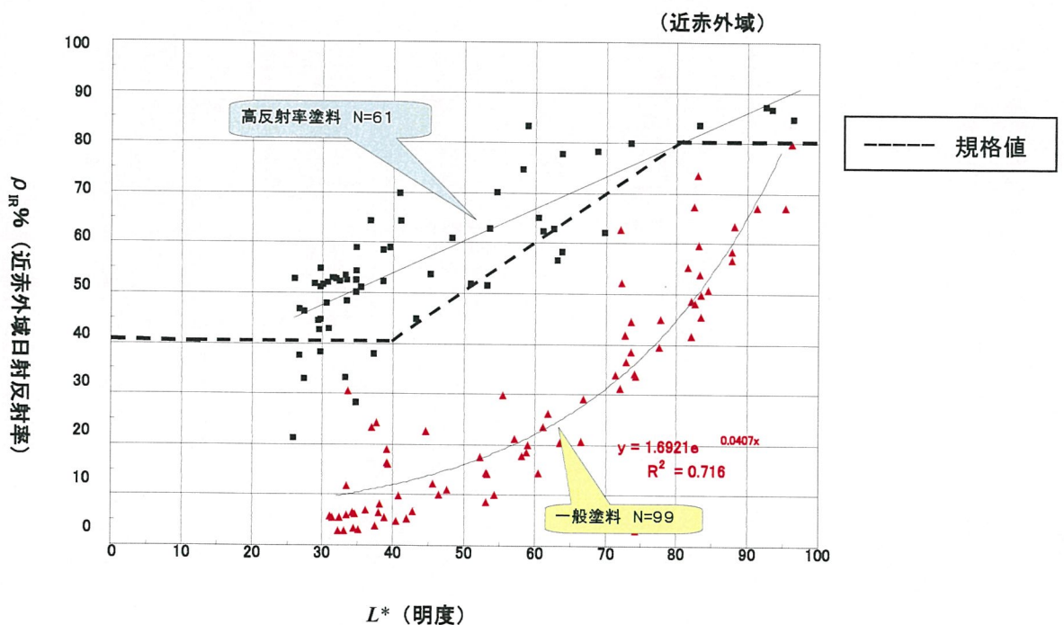
図1—明度(L*値)と近赤外域日射反射率(%)との関係
